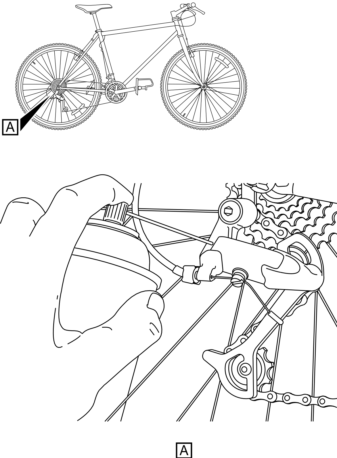
Fig 1 Derailleur pivots
