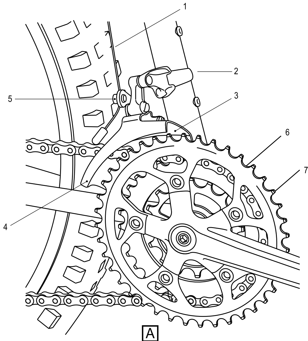
Fig 1 Front derailleur
